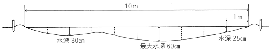
観察池の断面積
